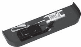
MusicZone Soundmodul, mit Bluetooth-Steuerung inkl. Körperschallwandler, 12V, 6W zur Montage unter Möbeln ab 450 mm Breite
