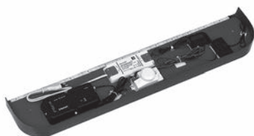
Light + MusicZone LED-Leuchte, mit Bewegungssensor und Sound-Modul mit Bluetooth-Steuerung, inkl. Körperschallwandler, 12V LED, LM LED, 10W zur Montage unter Möbeln ab 700 mm Breite
